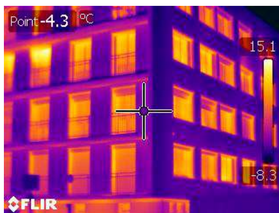
isolation par l'extérieur source ALEC42
